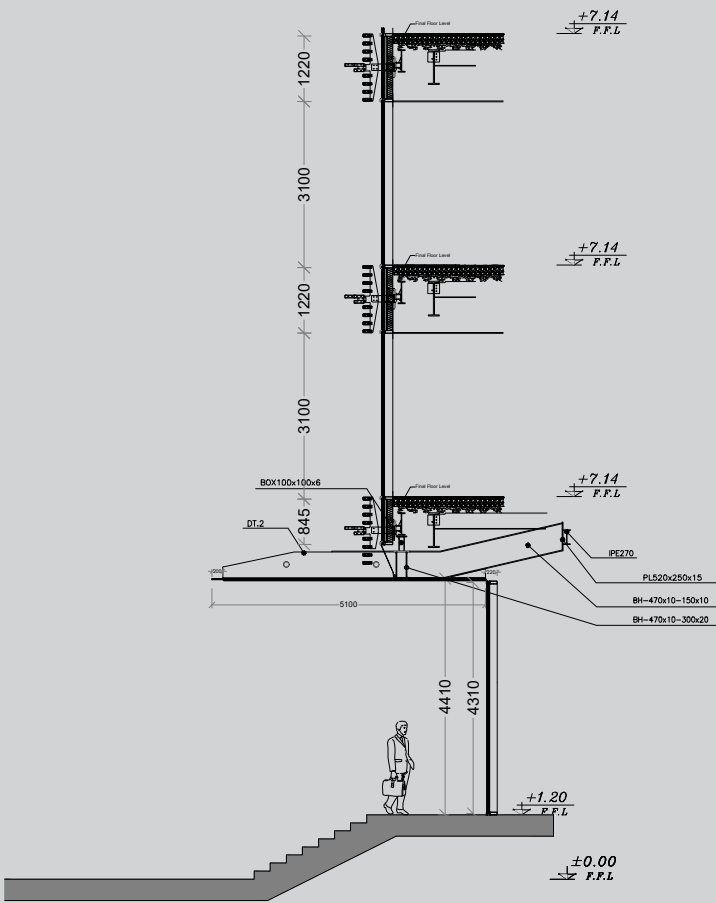
SECTION A-A
